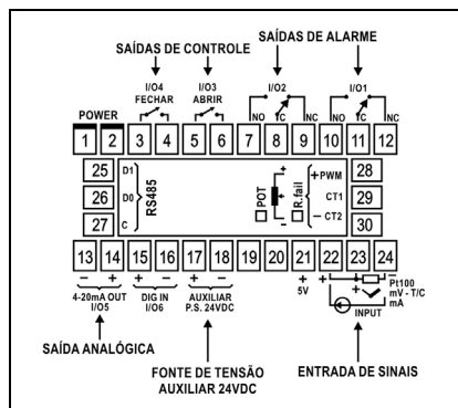
Figura 2 - Conexões do painel traseiro
