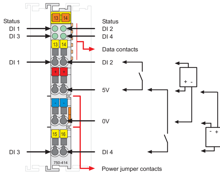
Fig. 2.1.1-1: View
