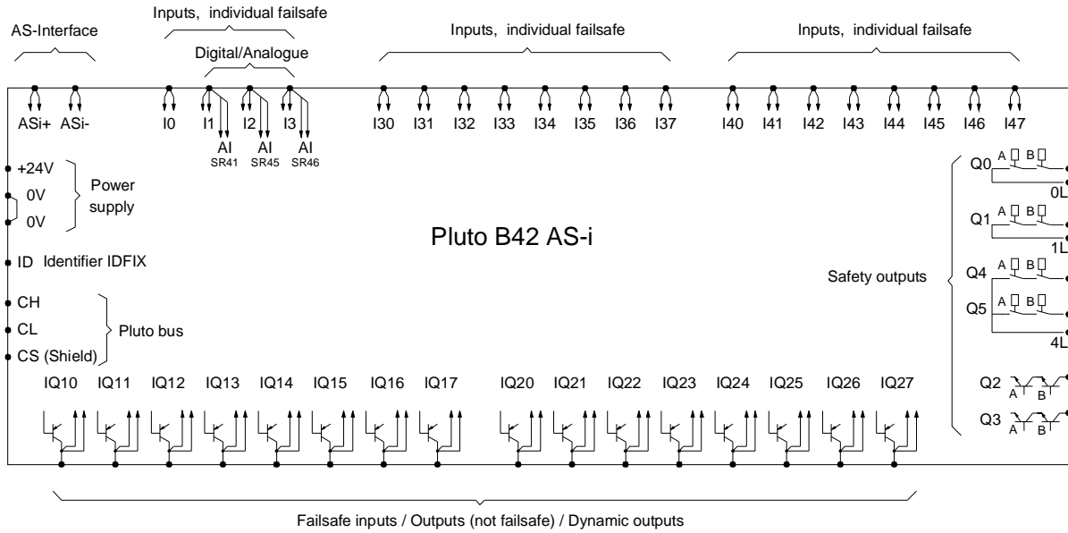
I/O overview PLUTO B42 AS-i
